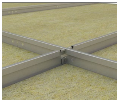
Bæreprøfiler og tverrprofiler har alle en høyde på 38 mm, som sikrer høy stabilitet og bedre integrasjonsmuligheter med armaturer.
